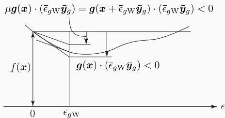
図 3.7: Wolfe の規準
