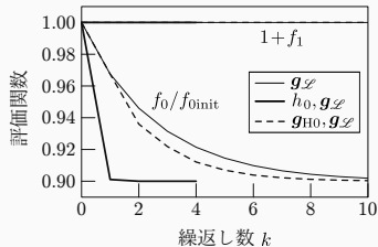
(a) 評価関数
