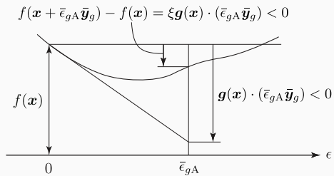
図 3.5: Armijo の規準
