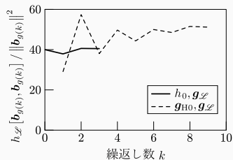
(e) 探索経路上 f_0 2 階微分 (f) 探索経路上 f_0 2 階微分 (探索距離)
