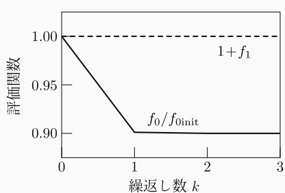
(b) 評価関数の履歴
