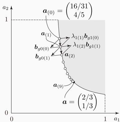
(a) 試行点の推移
