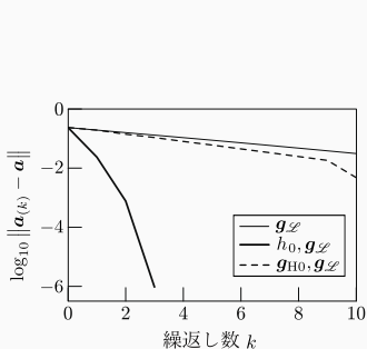
(a) 収束履歴
