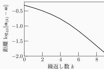
(c) 最小点からの距離 \|a_k - a\|_{\mathbb{R}^2}
