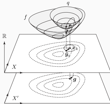
図 3.2: 勾配法
