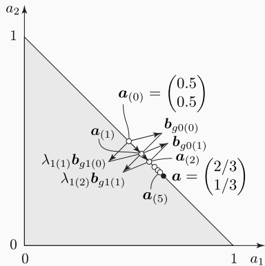
(a) 試行点の推移
