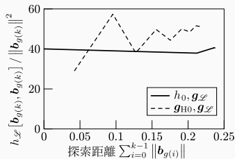
(e) 探索経路上 f_0 2 階微分 (f) 探索経路上 f_0 2 階微分 (探索距離)
