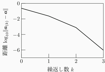
(c) 最小点からの距離 \|a_k - a\|_{\mathbb{R}^2}
