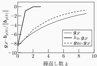
(c) 探索経路上 f_0 勾配
