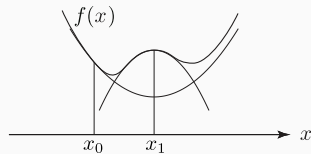
(b) 極大値に収束する場合
