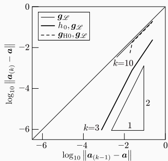
(b) (k-1) 回目対 k 回目の関係
