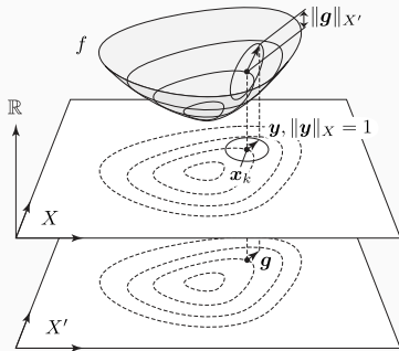
図 3.1: 勾配 g の定義
