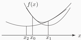
(a) 収束しない場合
