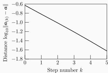
(c) 最小点からの距離 \|a_k - a\|_{\mathbb{R}^2}
