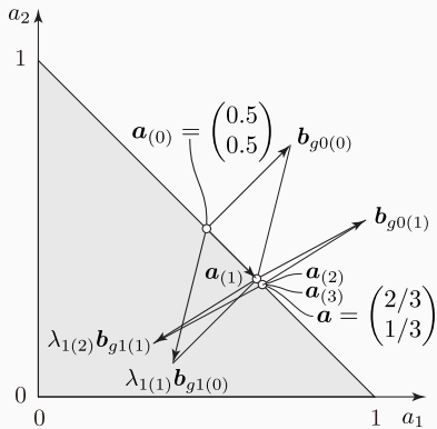
(a) 試行点の推移
