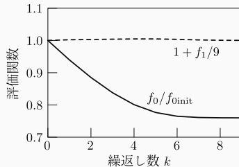
(b) 評価関数の履歴
