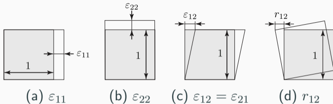
図 5.6: 2次元線形弾性体の線形ひずみ E(u) と回転テンソル R(u) の成分
