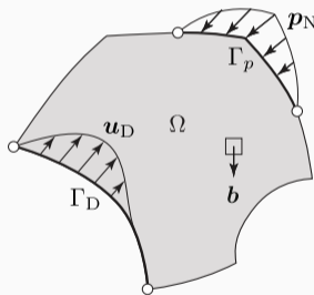
図 5.4: 線形弾性問題
