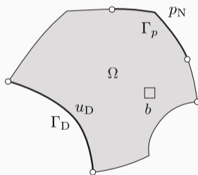
図 5.1: 領域 \Omega とその境界 \partial\Omega = \bar{\Gamma}_D \cup \bar{\Gamma}_N
