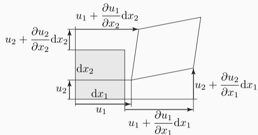
図 5.5: 2次元線形弾性体の変位 u と変位勾配 (\nabla u^\top)^\top の成分
