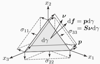
図 5.8: 3次元線形弾性体の Cauchy 応力 S と応力 p
