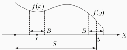
図 2.7: 関数 f の極小点 x と最小点 y
