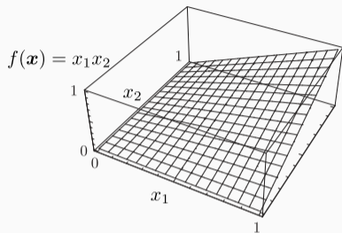
図 2.13: 関数 f(\mathbf{x}) = x_1x_2
