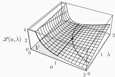
図 2.25: 例題 2.9.4 の鞍点
