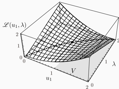
図 2.23: 例題 2.9.3 の鞍点
