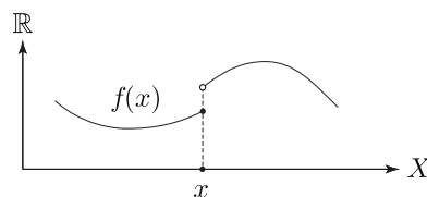
図 A.1.3: 関数の下半連続性
