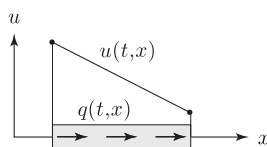
図 A.6.2: Fourier の熱伝導法則
