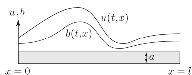
図 A.6.1: 1次元熱伝導問題
