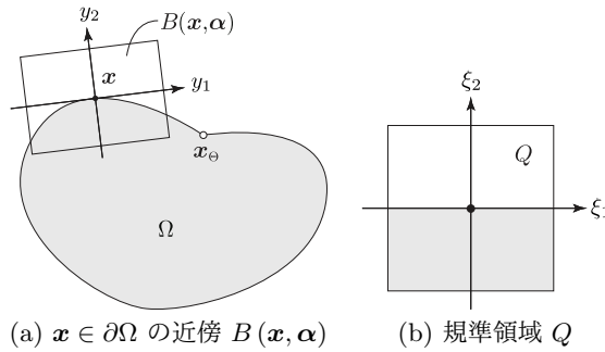
図 A.5.3: 区分的 C^1 級境界
