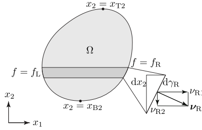
図 A.8.1: Gauss の発散定理
