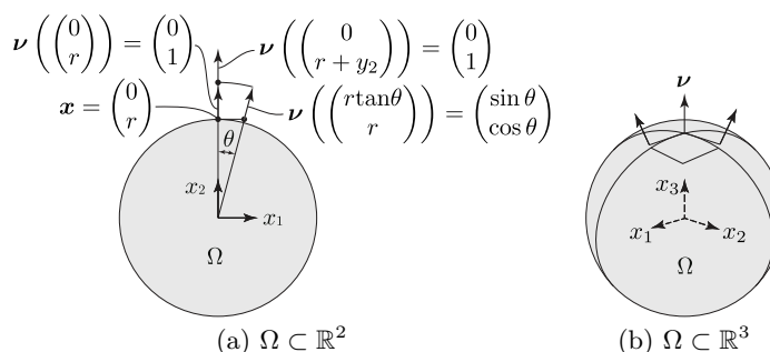
図 A.5.6: 円と球の平均曲率
