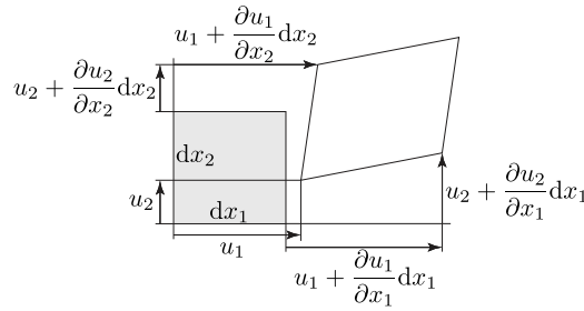
図 5.4.2: 2次元線形弾性体の変位 \mathbf{u} と変位勾配 (\nabla \mathbf{u}^\top)^\top の成分
