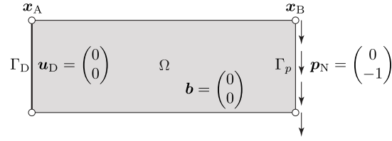
図 5.8.1: 線形弾性体の片持ちはり問題
