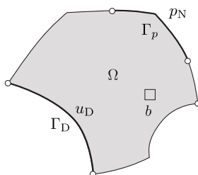
図 5.1.1: 領域 \Omega とその境界 \partial\Omega = \bar{\Gamma}_D \cup \bar{\Gamma}_N
