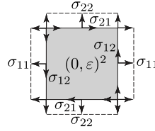
図 5.4.6: 2次元線形弾性体の微小面積におけるモーメントのつり合い ( \epsilon \ll 1 )
