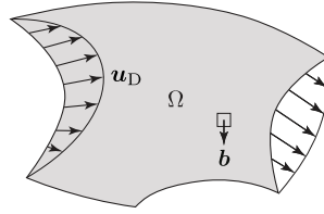
図 5.5.1: Stokes 問題
