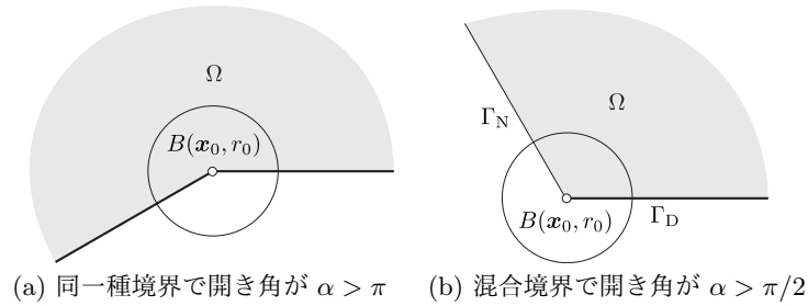
図 5.3.2: 特異性が現れる角をもつ 2 次元領域
