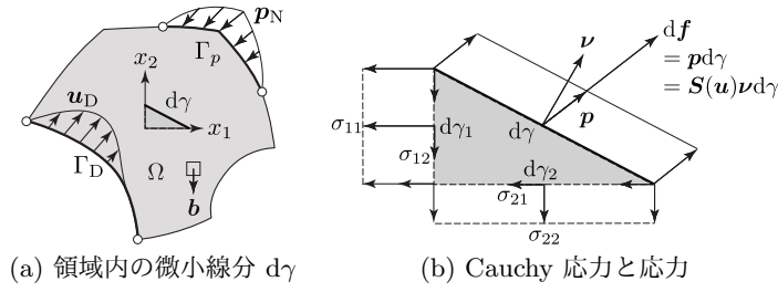
図 5.4.4: 2次元線形弾性体の Cauchy 応力 S と応力 p
