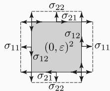
図 5.4.6: 2次元線形弾性体の微小面積におけるモーメントのつり合い ( \epsilon \ll 1 )
