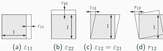
図 5.4.3: 2次元線形弾性体の線形ひずみ E(u) と回転テンソル R(u) の成分
