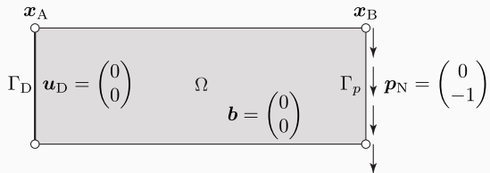
図 5.8.1: 線形弾性体の片持ちはり問題
