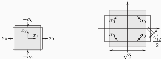
(a) 圧縮と引張 (b) 反時計回りに \pi/4 だけ回転した座標系
