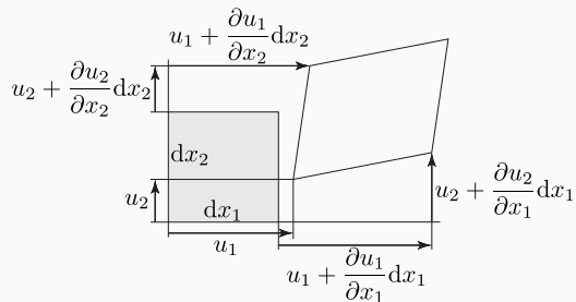
図 5.4.2: 2次元線形弾性体の変位 u と変位勾配 (\nabla u^T)^T の成分
