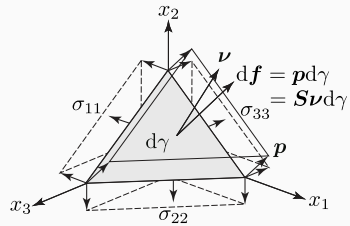
図 5.4.5: 3次元線形弾性体の Cauchy 応力 S と応力 p
