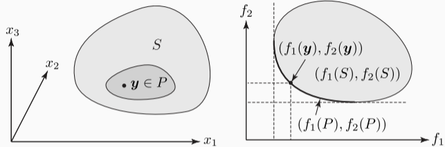
(a) 設計変数の線形空間 (b) 評価関数の線形空間
