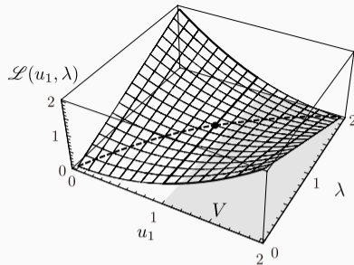
図 2.9.2: 例題 2.9.3 の鞍点
