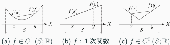
図 2.4.3: f が凸関数の例 ( X = \mathbb{R} )
