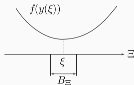
(b) \xi 座標系
