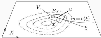
(a) \xi - u 座標系
