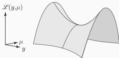
図 2.9.1: 鞍点
