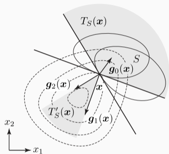
図 2.7.2: X = \mathbb{R}^2 および m = 2 のときの不等式制約つき最適化問題における極小点
