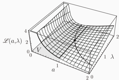
図 2.9.4: 例題 2.9.4 の鞍点
