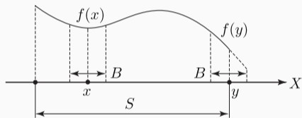
図 2.3.1: 関数 f の極小点 x と最小点 y
