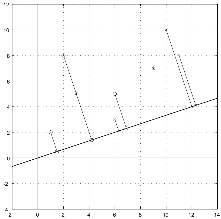
図 2: (m_1 - m_2) の軸への射影
