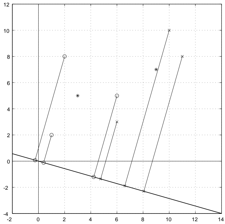
図 1: Fisher の軸への射影
